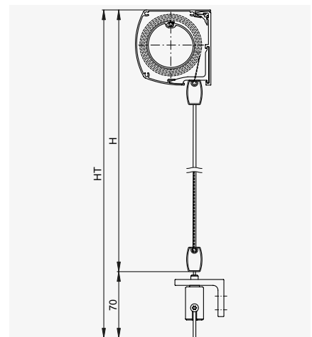
Guidage câbles
